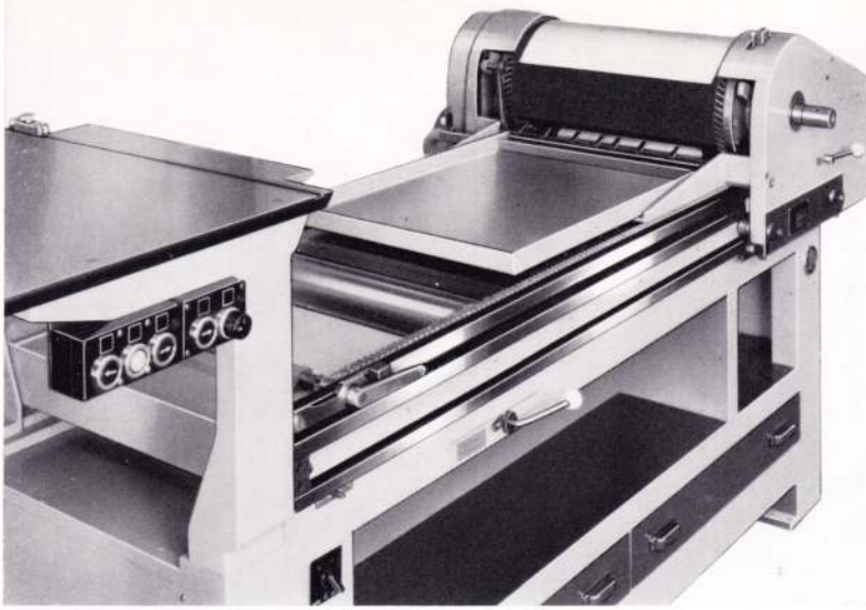
Druckzylinder in Endstellung
