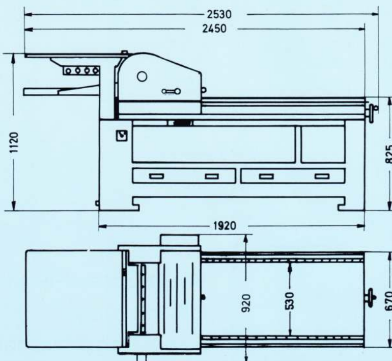
Hauptabmessungen
