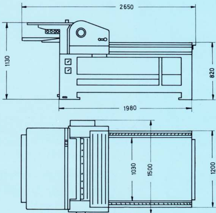
Hauptabmessungen
