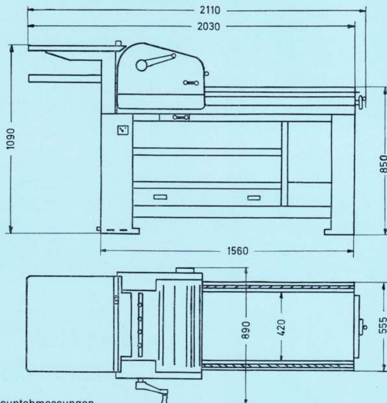
Hauptabmessungen
