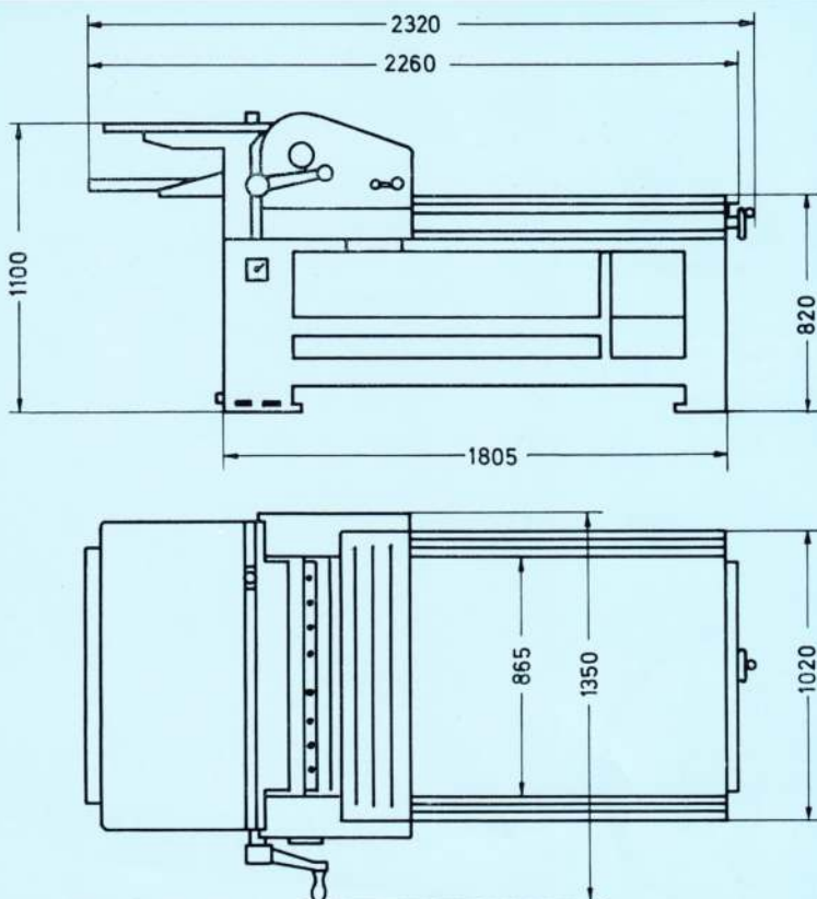
Hauptabmessungen
