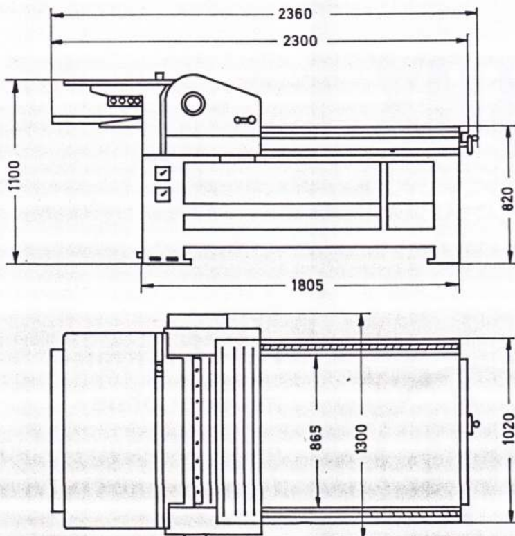
Hauptabmessungen
