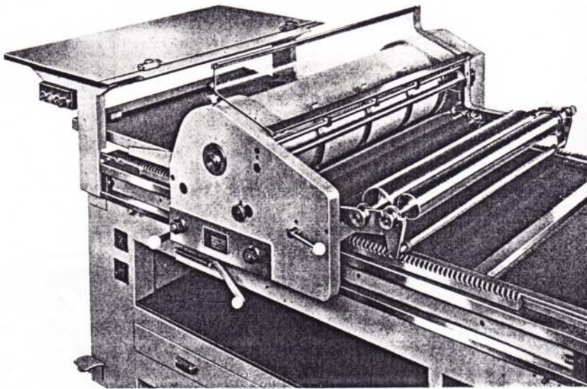
Farbwerk durch Aufklappen bequem zugänglich
