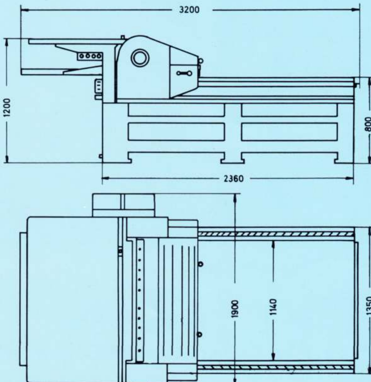
Hauptabmessungen
