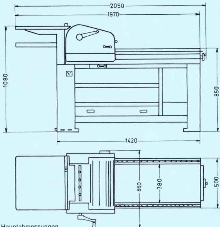
Hauptabmessungen
