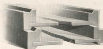
Detail van de afwerking der zijkanen, waardoor de stapel onwrikbaar is
